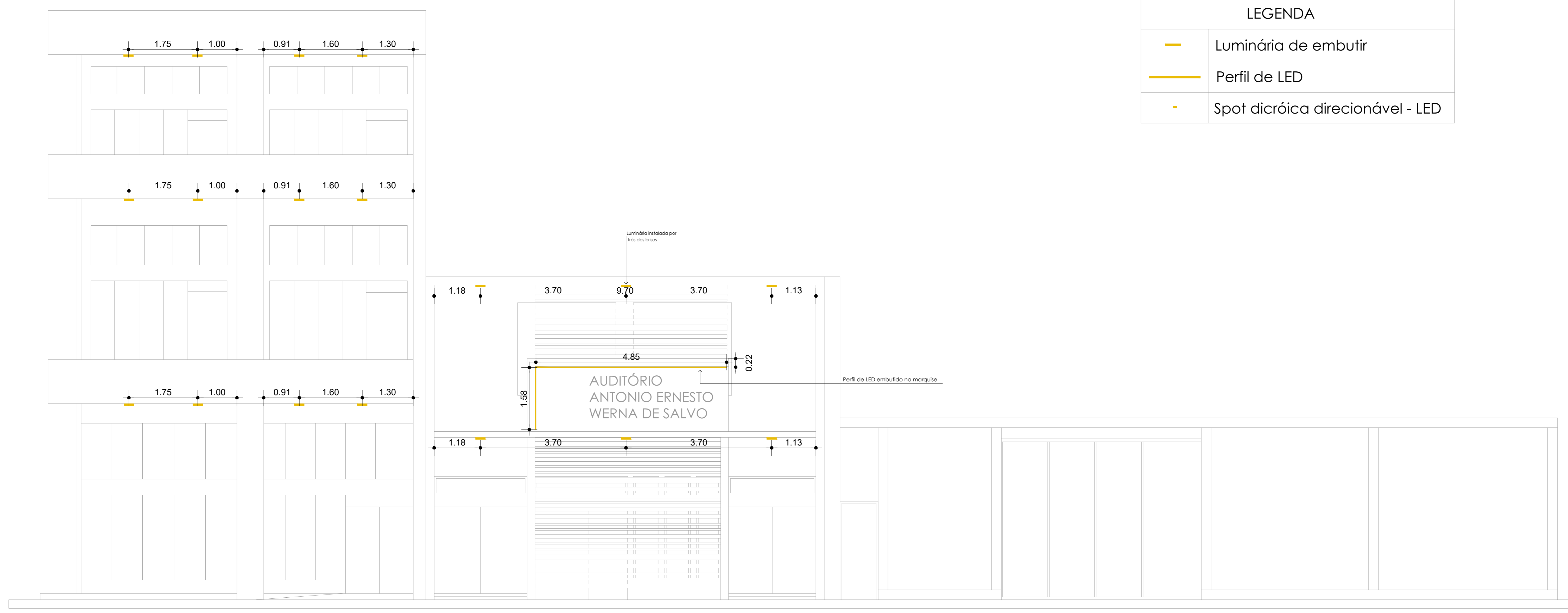
LOCAÇÃO PONTOS DE ILUMINAÇÃO - FACHADA LATERAL Projeto Institucional ESCALA: 1/50
