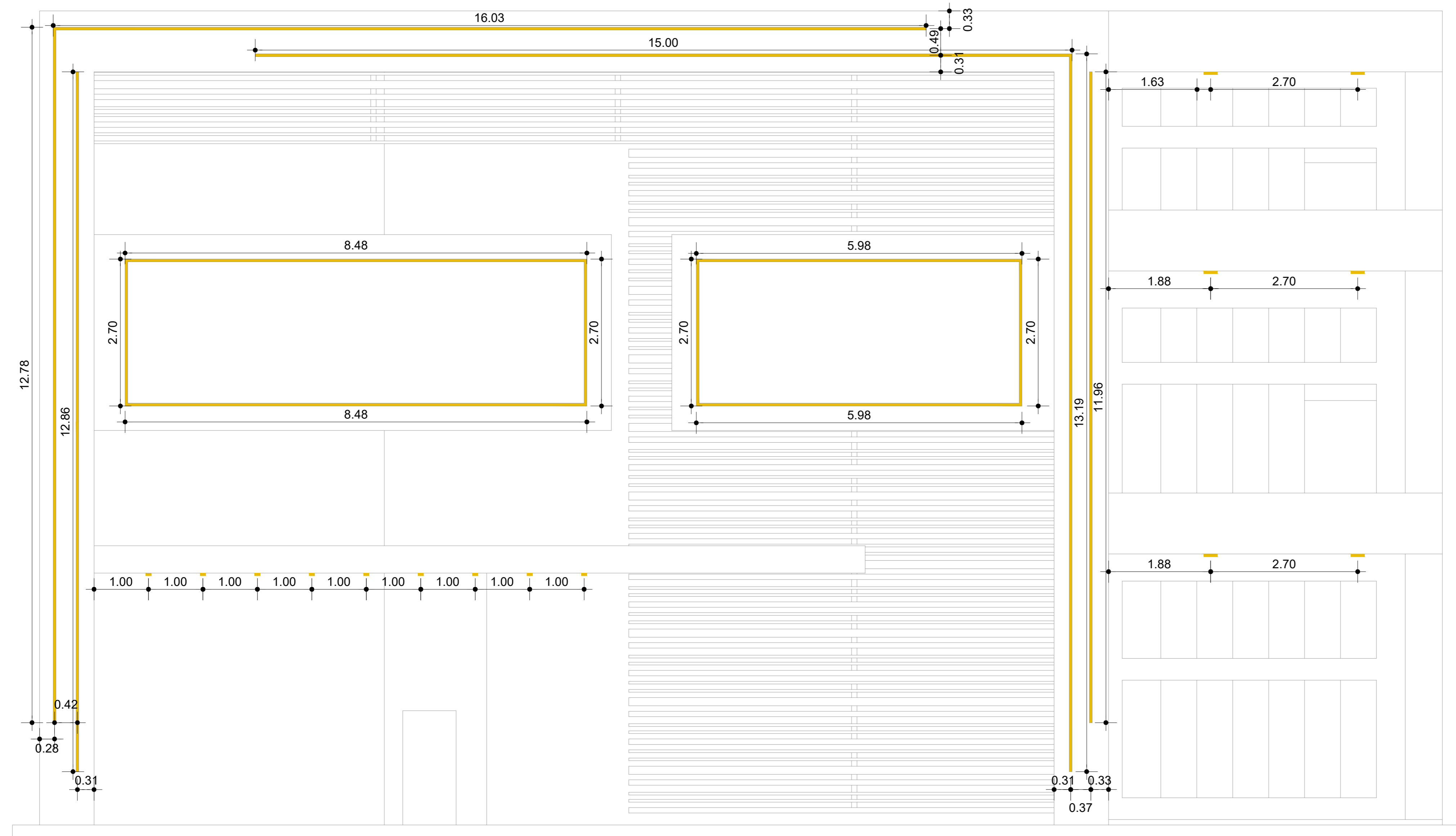
LOCAÇÃO PONTOS DE ILUMINAÇÃO - FACHADA FRONTAL Projeto Institucional ESCALA: 1/50
