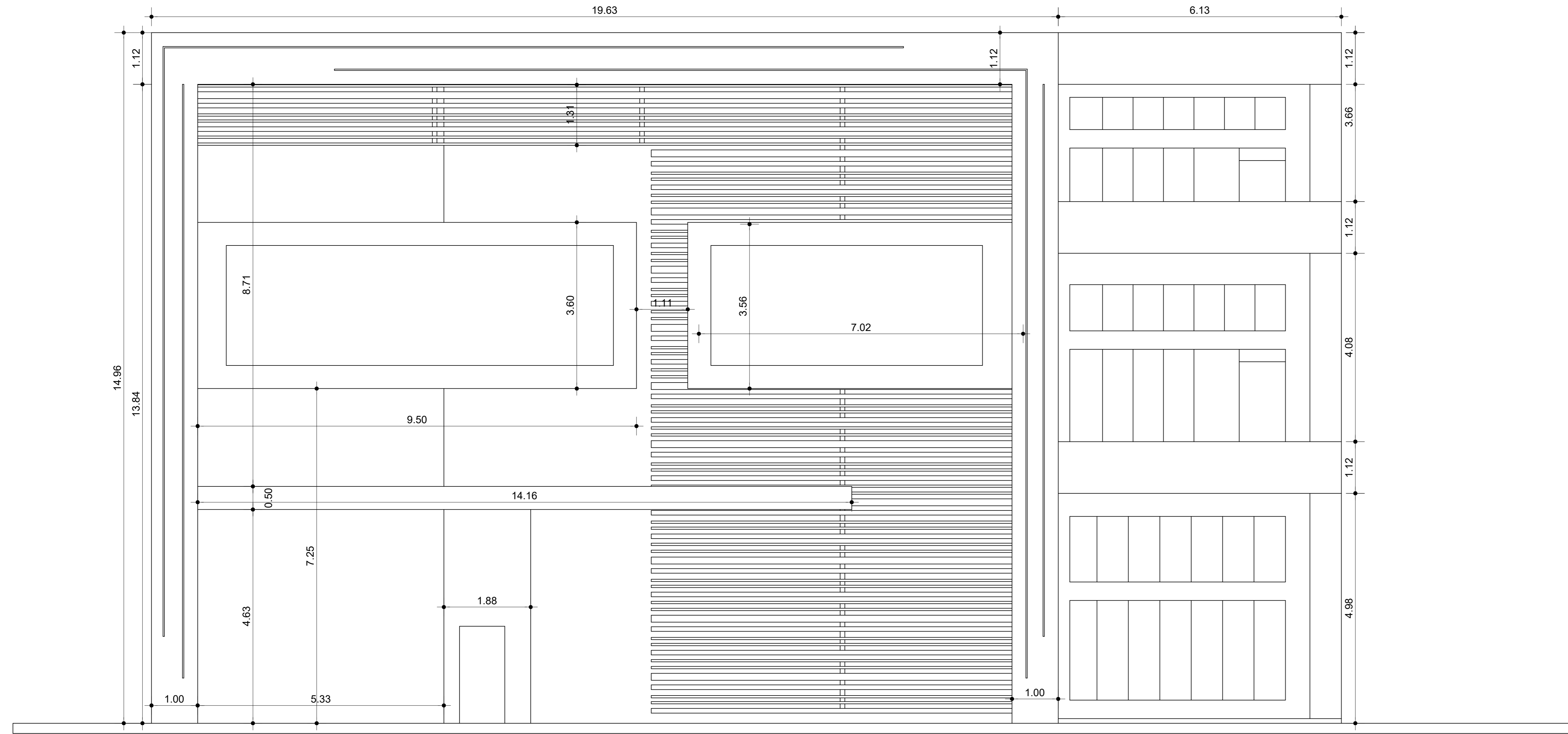
VISTA FACHADA FRONTAL Projeto Institucional ESC. 1/50
