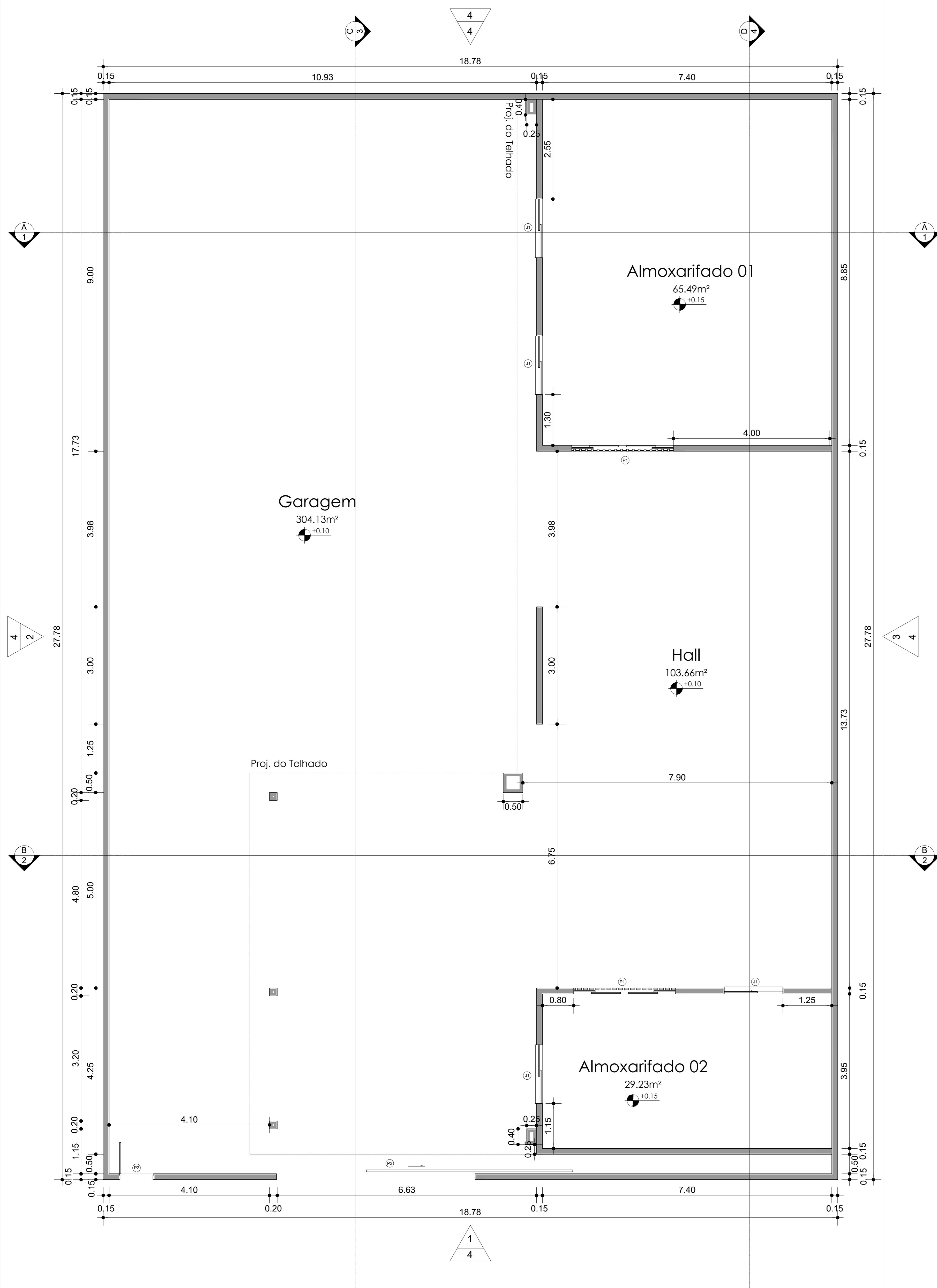
PLANTA BAIXA COTADA Projeto Institucional ESC. 1/50
